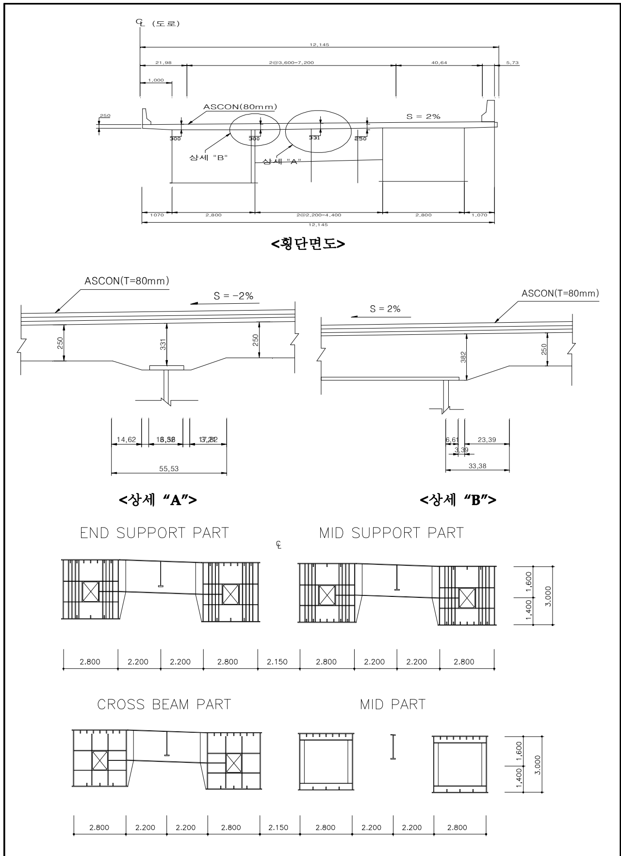
【그림 1.4】 횡단면도
